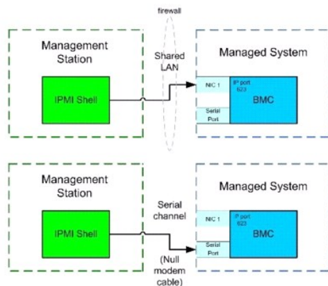
Figure 3-2. Schéma de l'environnement IPMI
